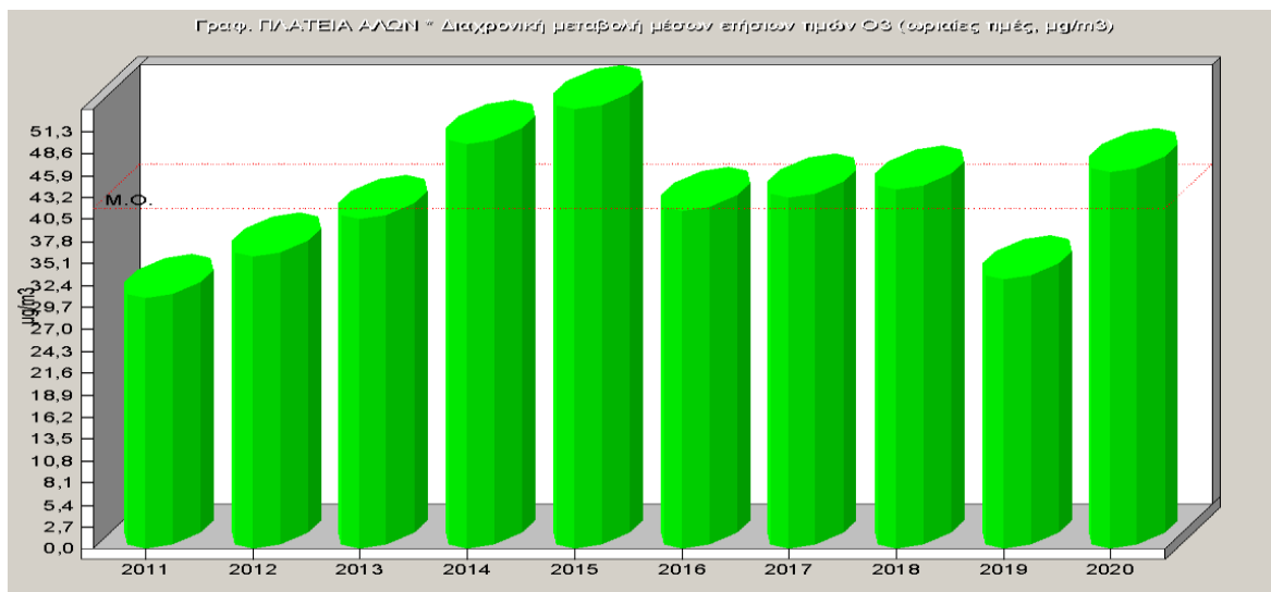
Σχήμα 2.4. Μέσες ετήσιες τιμές όζοντος 2011-2020.
