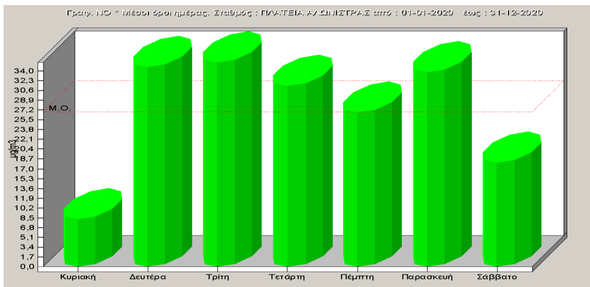
Σχήμα 2.12: Ημερήσια μεταβολή των συγκεντρώσεων μονοξειδίου του αζώτου για το έτος 2020.
