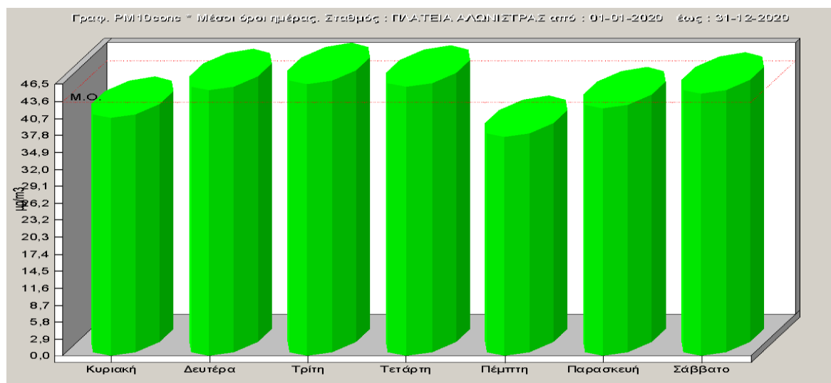
Σχήμα 2.15: Ημερήσια μεταβολή των συγκεντρώσεων αιωρούμενων σωματιδίων για το έτος 2020.
