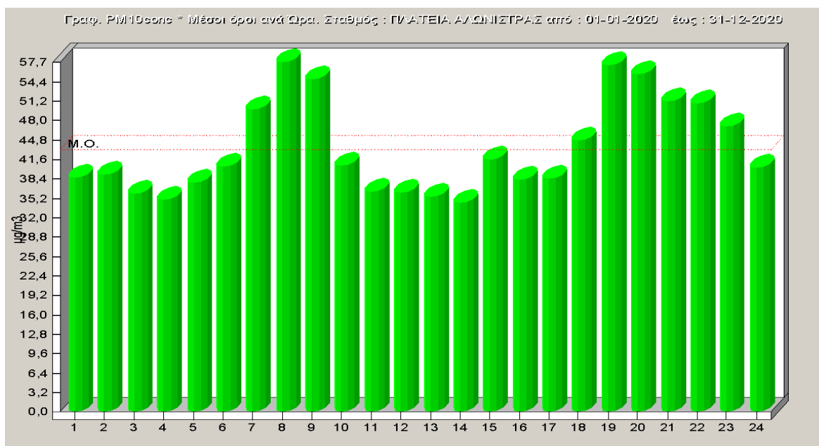
Σχήμα 2.20: Ωριαία μεταβολή αιωρούμενων σωματιδίων για το έτος 2020.
