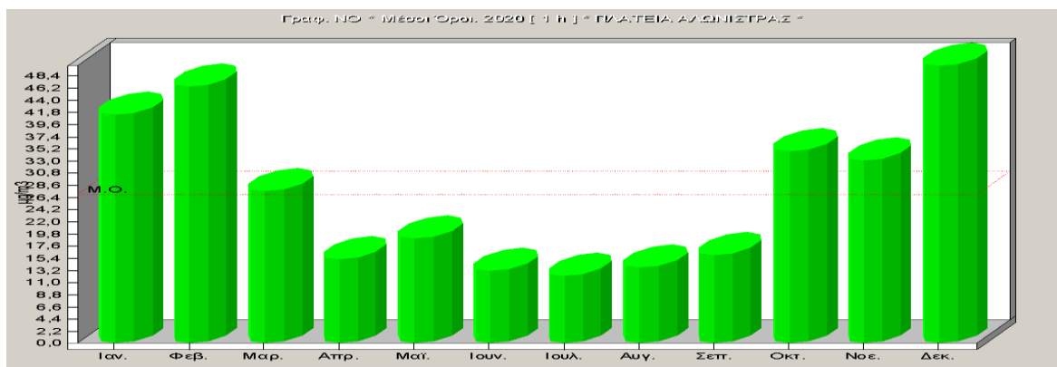
Σχήμα 2.7. Μέσες μηνιαίες τιμές μονοξειδίου του αζώτου για το έτος 2020.
