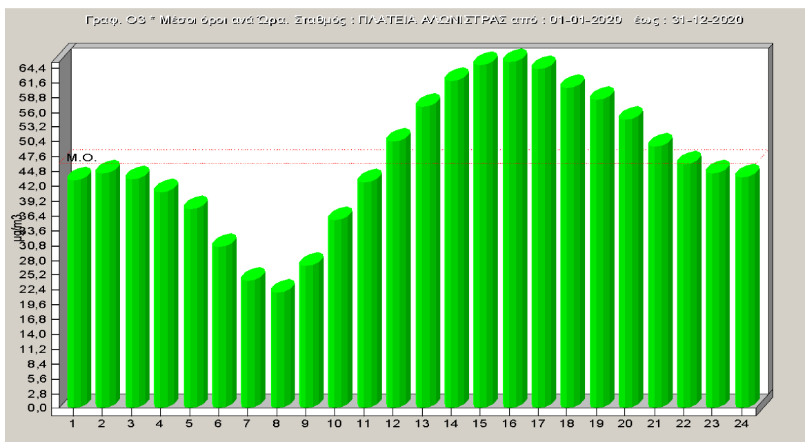
Σχήμα 2.19: Ωριαία μεταβολή όζοντος για το έτος 2020
