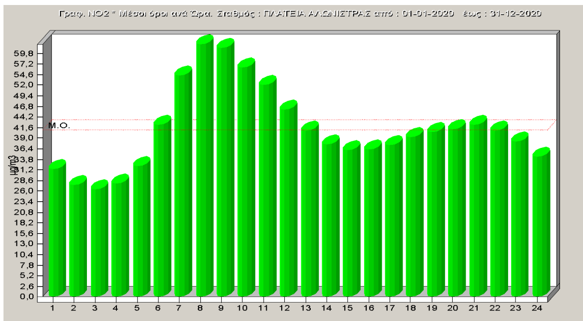
Σχήμα 2.18: Ωριαία μεταβολή διοξειδίου του αζώτου για το έτος 2020
