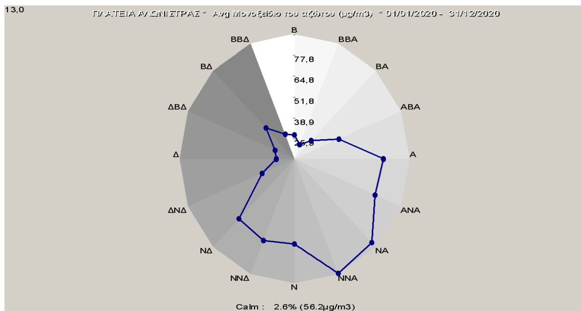
Σχήμα 3.5.: Μέσες τιμές μονοξειδίου του αζώτου, για κάθε διεύθυνση του ανέμου (σε \mu\text{g}/\text{m}^3 ), για το έτος 2020.
