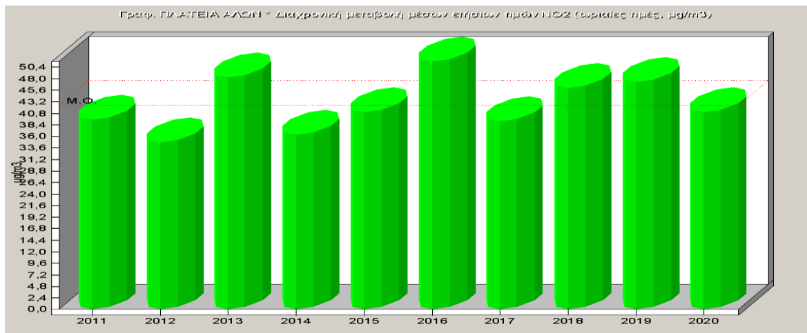
Σχήμα 2.3. Μέσες ετήσιες τιμές διοξειδίου του αζώτου 2011-2020.
