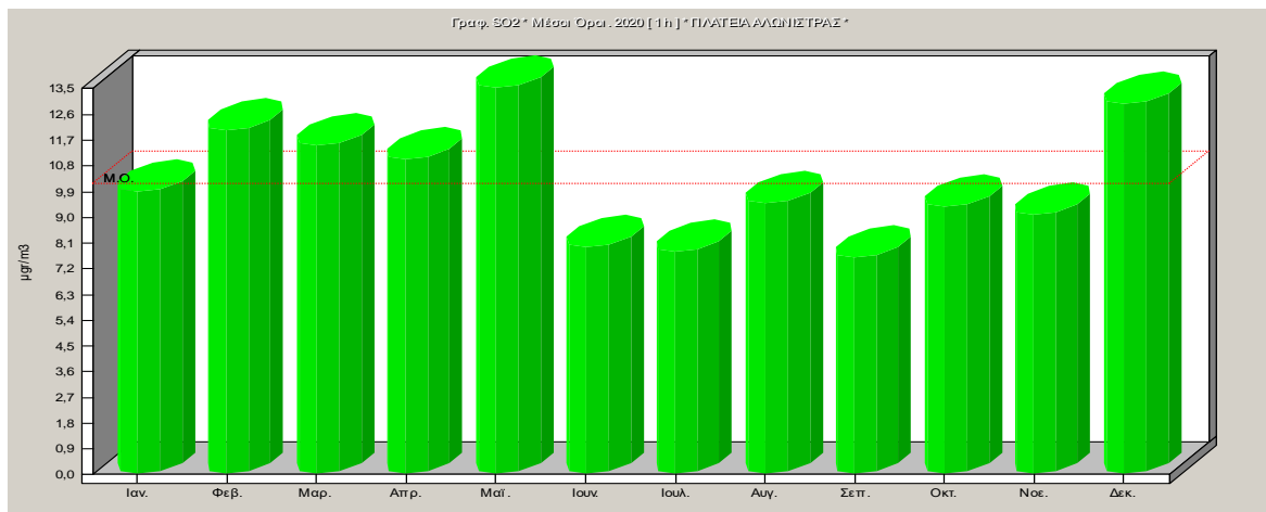
Σχήμα 2.6. Μέσες μηνιαίες τιμές διοξειδίου του θείου για το έτος 2020.
