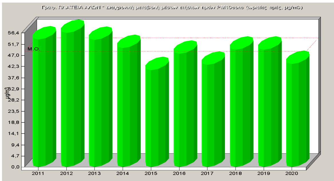
Σχήμα 2.5. Μέσες ετήσιες τιμές αιωρούμενων σωματιδίων 2011-2020.
