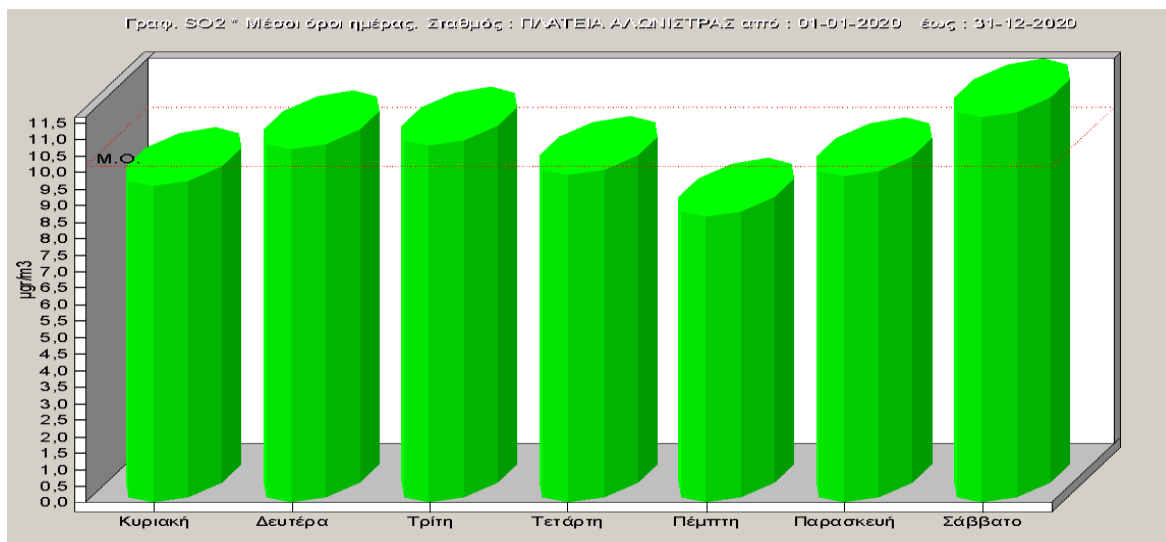
Σχήμα 2.11: Ημερήσια μεταβολή των συγκεντρώσεων διοξειδίου του θείου για το έτος 2020.
