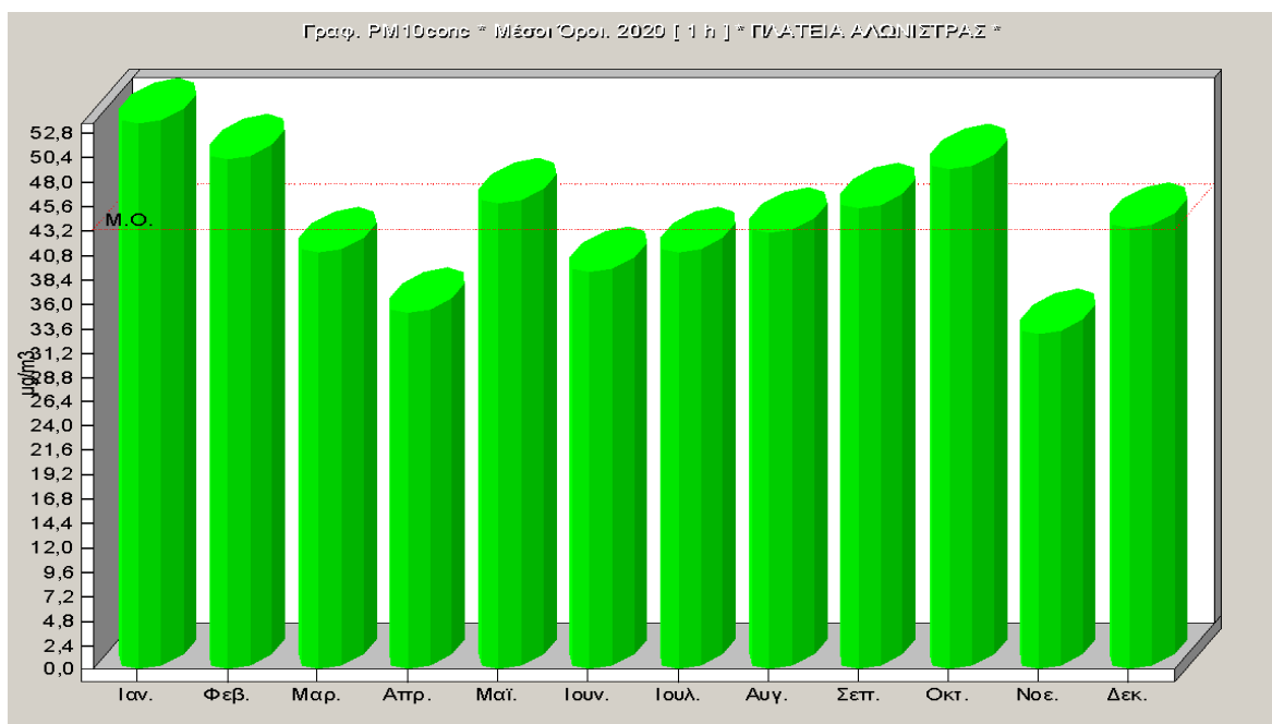
Σχήμα 2.10. Μέσες μηνιαίες τιμές αιωρούμενων σωματιδίων για το έτος 2020.
