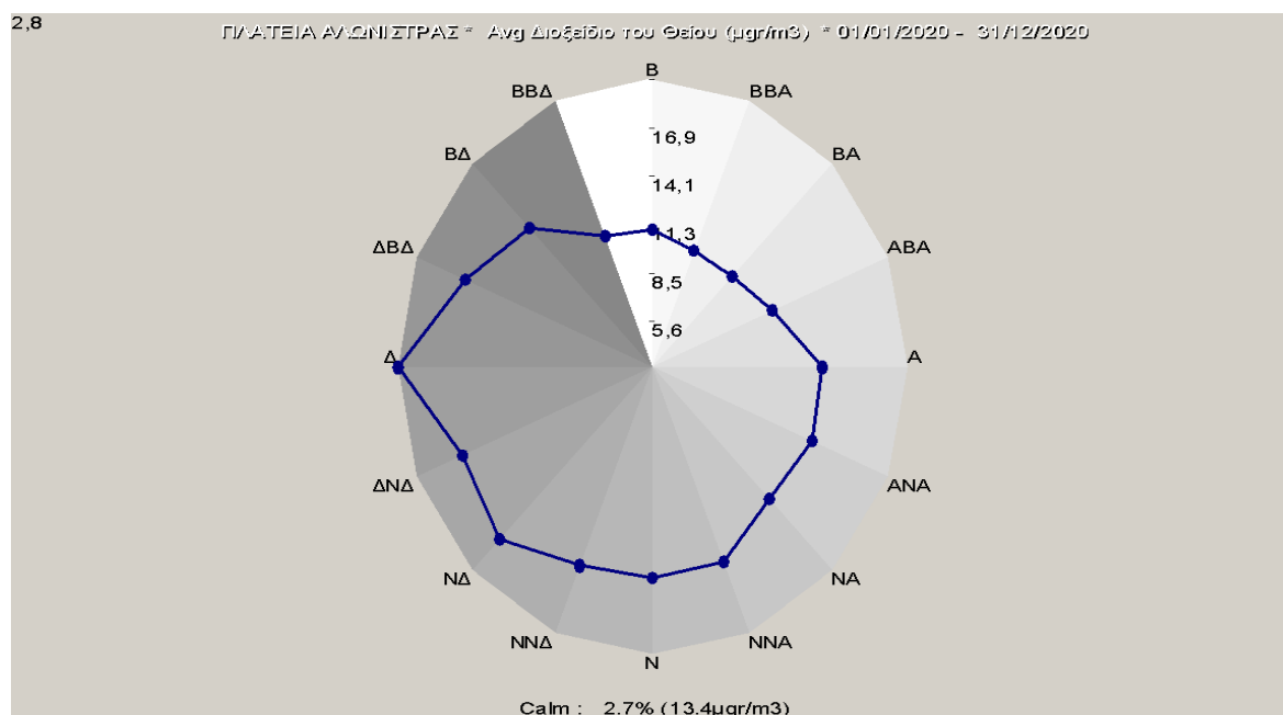
Σχήμα 3.3.: Μέσες τιμές διοξειδίου του θείου (σε \mu\text{g}/\text{m}^3 ), για κάθε διεύθυνση του ανέμου, για το έτος 2020.
