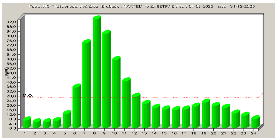
Σχήμα 2.17: Ωριαία μεταβολή μονοξειδίου του αζώτου για το έτος 2020
