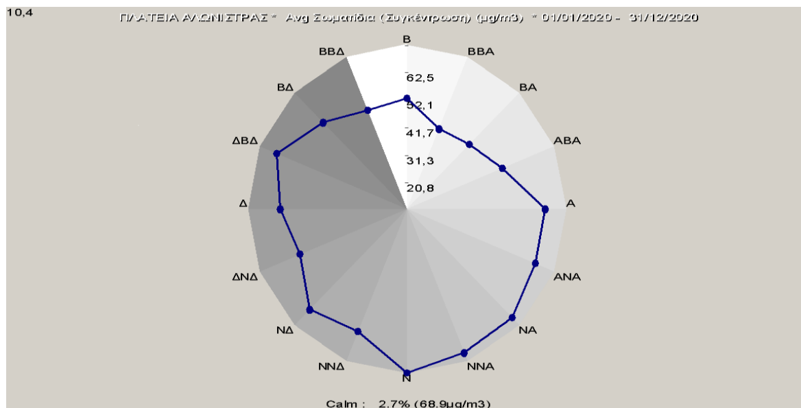
Σχήμα 3.7.: Μέσες τιμές Αιωρούμενων Σωματιδίων (σε \mu\text{g}/\text{m}^3 ), για κάθε διεύθυνση του ανέμου, για το έτος 2020.
