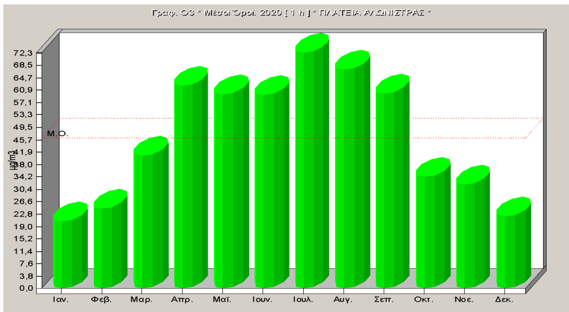
Σχήμα 2.9. Μέσες μηνιαίες τιμές όζοντος για το έτος 2020.
