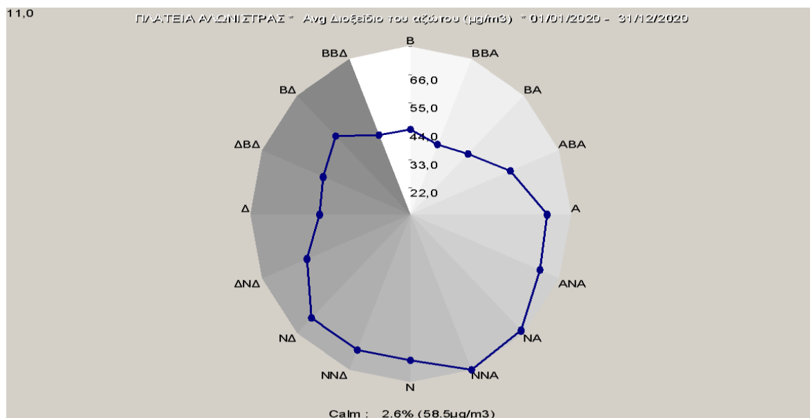
Σχήμα 3.6.: Μέσες τιμές διοξειδίου του αζώτου (σε \mu\text{g}/\text{m}^3 ), για κάθε διεύθυνση του ανέμου, για το έτος 2020.
