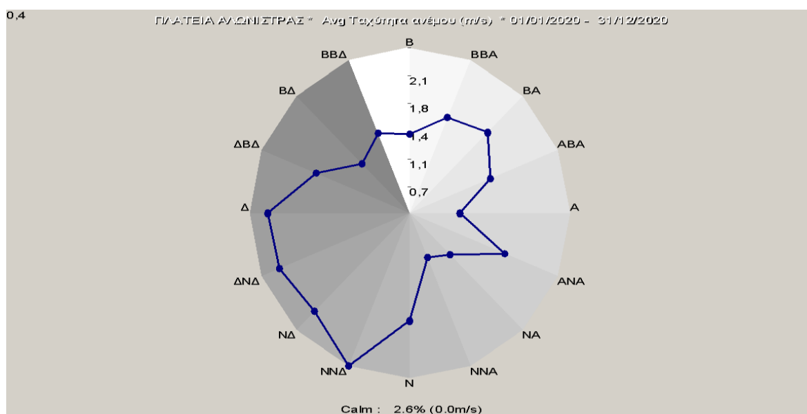
Σχήμα 3.2 Μέση ταχύτητα ανά διεύθυνση ανέμου, για το έτος 2020.
