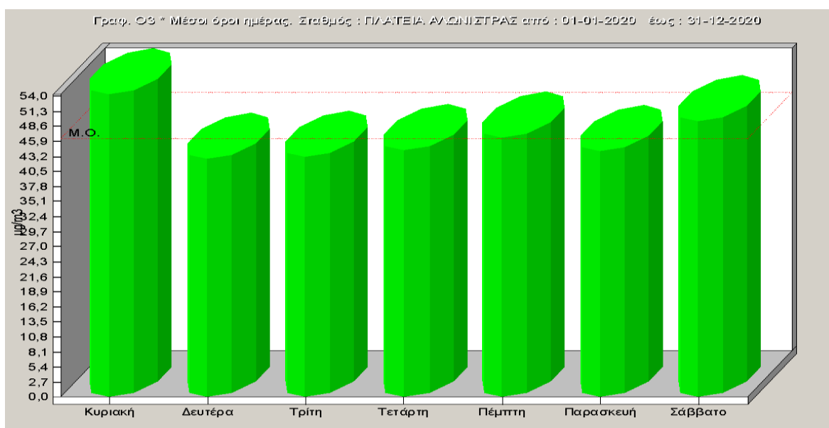
Σχήμα 2.14: Ημερήσια μεταβολή των συγκεντρώσεων όζοντος για το έτος 2020.
