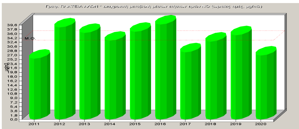
Σχήμα 2.2. Μέσες ετήσιες τιμές μονοξειδίου του αζώτου 2011-2020.
