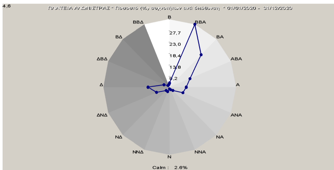
Σχήμα 3.1. Συχνότητες, επί τοις εκατό (%) των διευθύνσεων του ανέμου για το έτος 2020.
