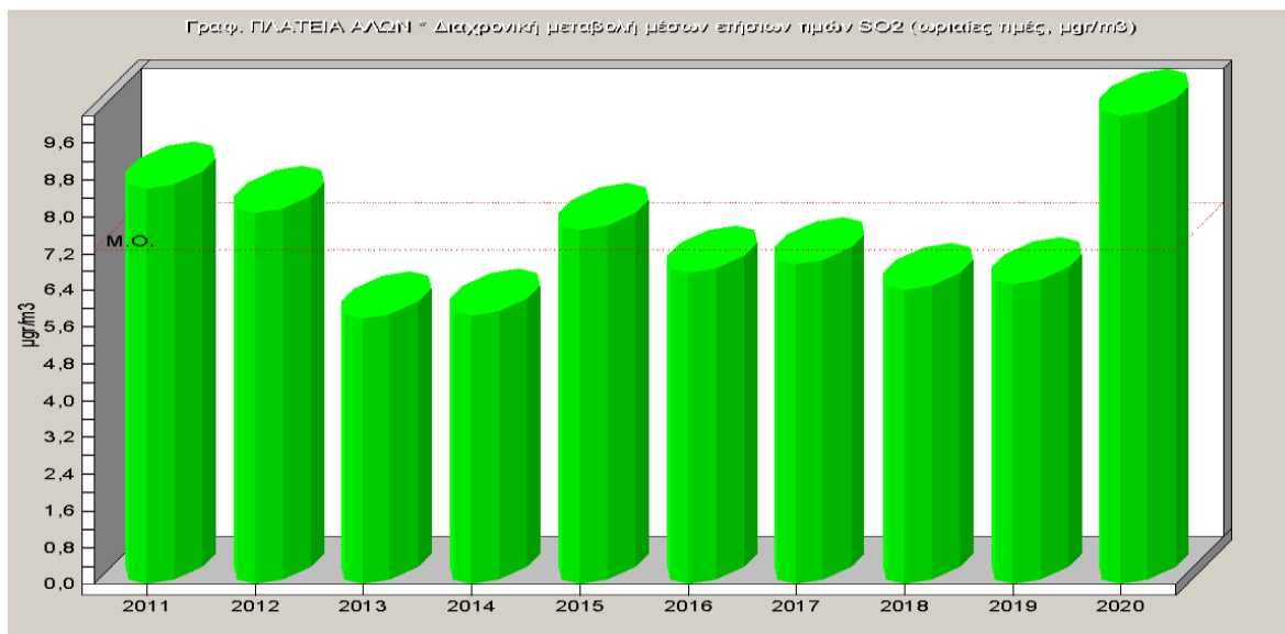
Σχήμα 2.1. Μέσες ετήσιες τιμές διοξειδίου του θείου 2011-2020.
