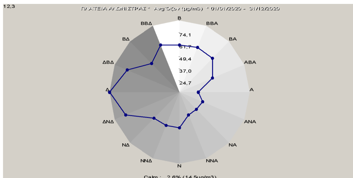
Σχήμα 3.4.: Μέσες τιμές όζοντος (σε \mu\text{g}/\text{m}^3 ), για κάθε διεύθυνση του ανέμου, για το έτος 2020.
