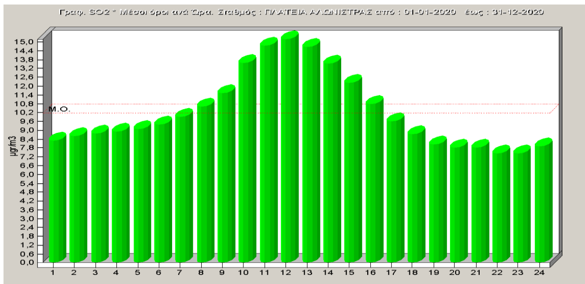
Σχήμα 2.16: Ωριαία μεταβολή διοξειδίου του θείου για το έτος 2020
