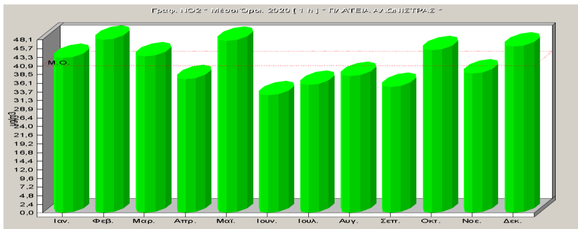
Σχήμα 2.8. Μέσες μηνιαίες τιμές διοξειδίου του αζώτου για το έτος 2020.
