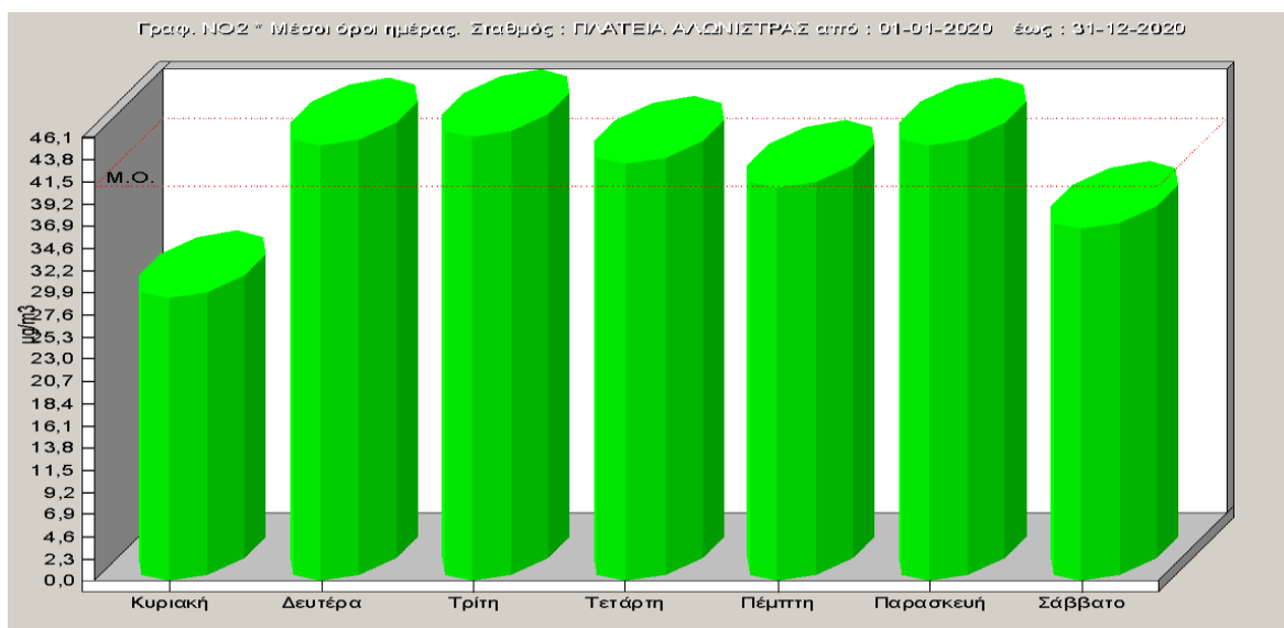
Σχήμα 2.13: Ημερήσια μεταβολή των συγκεντρώσεων διοξειδίου του αζώτου για το έτος 2020.
