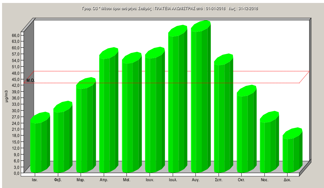
Σχήμα 2.9. Μέσες μηνιαίες τιμές όζοντος για το έτος 2018.
