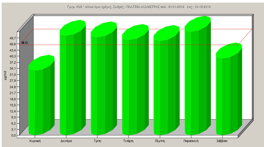
Σχήμα 2.13: Ημερήσια μεταβολή των συγκεντρώσεων διοξειδίου του αζώτου για το έτος 2018.
