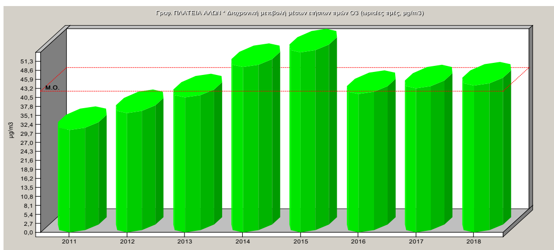
Σχήμα 2.4. Μέσες ετήσιες τιμές όζοντος 2011-2018.
