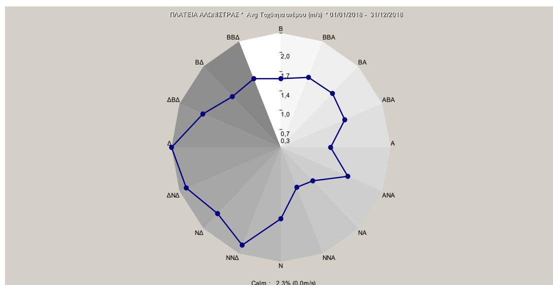
Σχήμα 3.2 Μέση ταχύτητα ανά διεύθυνση ανέμου, για το έτος 2018.
