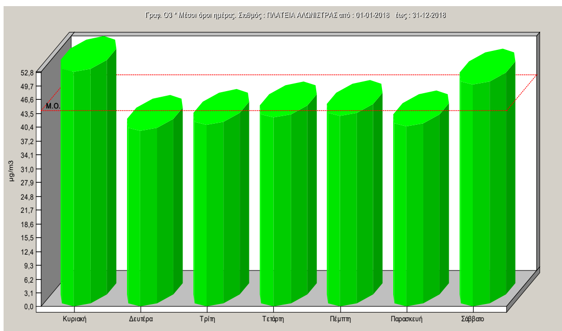
Σχήμα 2.14: Ημερήσια μεταβολή των συγκεντρώσεων όζοντος για το έτος 2018.
