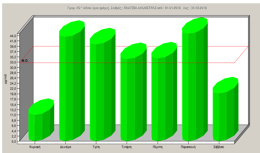
Σχήμα 2.12: Ημερήσια μεταβολή των συγκεντρώσεων μονοξειδίου του αζώτου για το έτος 2018.
