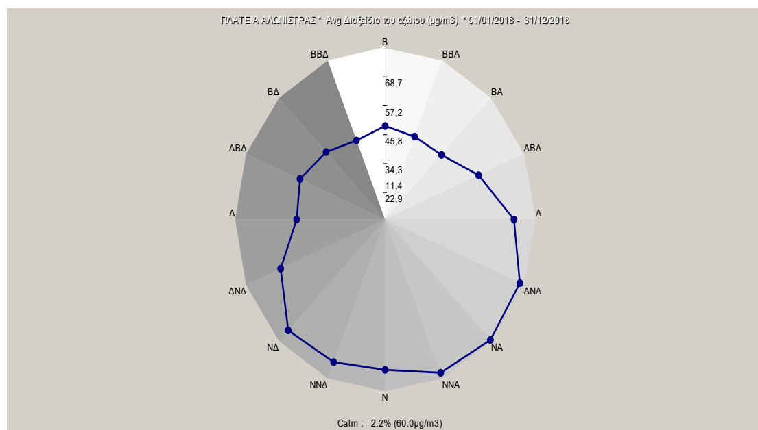
Σχήμα 3.6.: Μέσες τιμές διοξειδίου του αζώτου (σε \mu\text{g}/\text{m}^3 ), για κάθε διεύθυνση του ανέμου, για το έτος 2018.
