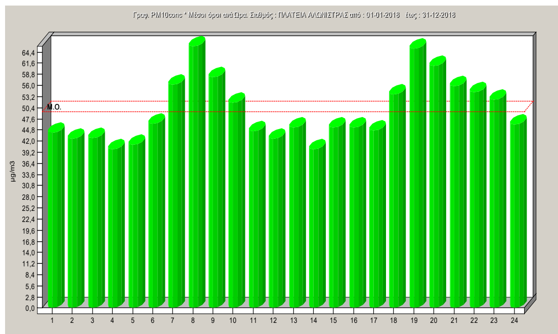
Σχήμα 2.20: Ωριαία μεταβολή αιωρούμενων σωματιδίων για το έτος 2018
