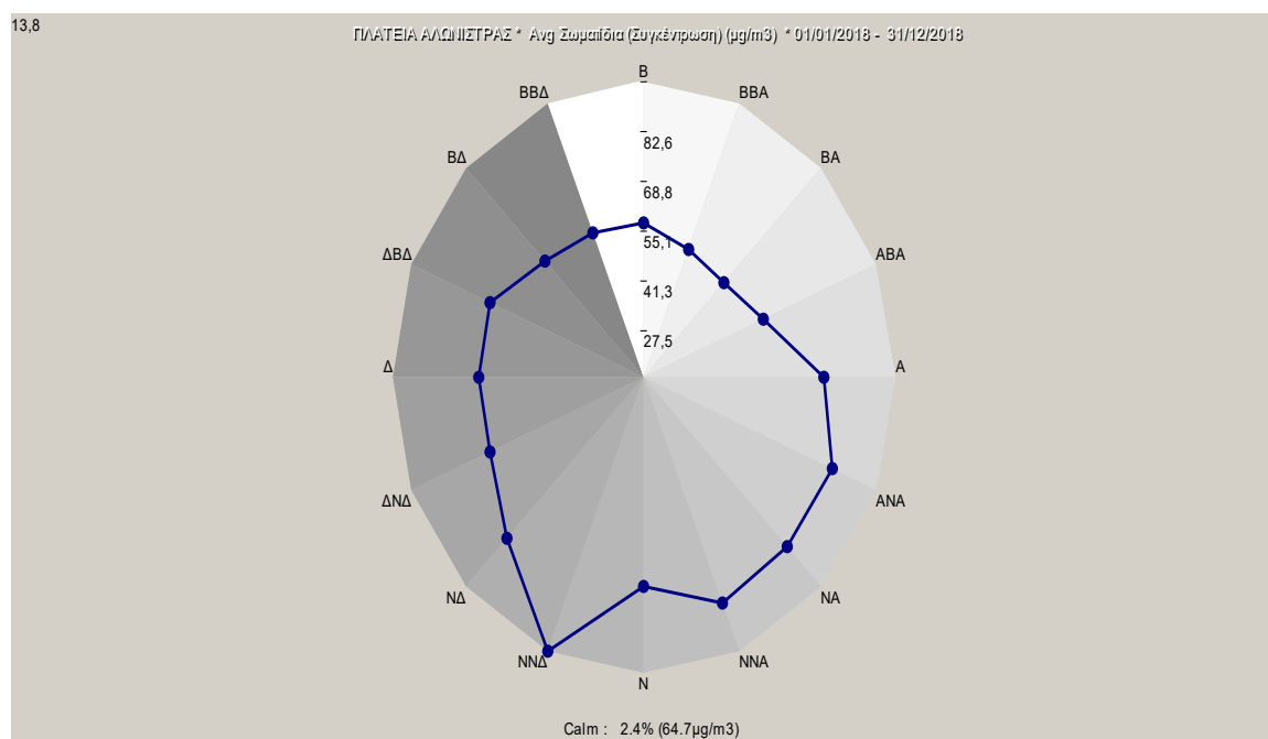
Σχήμα 3.7.: Μέσες τιμές Αιωρούμενων Σωματιδίων (σε \mu\text{g}/\text{m}^3 ), για κάθε διεύθυνση του ανέμου, για το έτος 2018.
