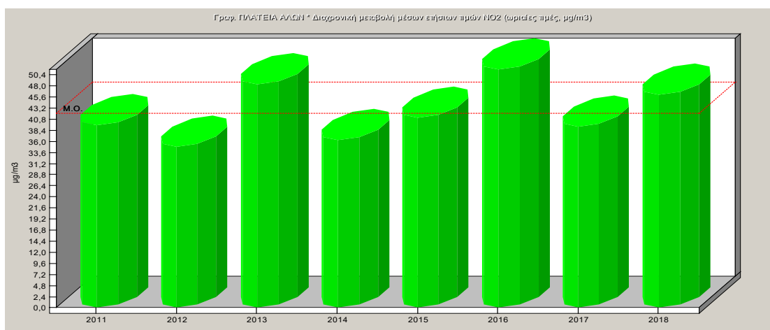
Σχήμα 2.3. Μέσες ετήσιες τιμές διοξειδίου του αζώτου 2011-2018.
