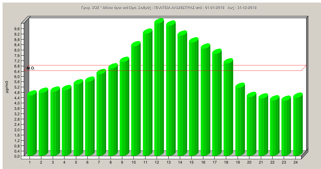
Σχήμα 2.16: Ωριαία μεταβολή διοξειδίου του θείου για το έτος 2018
