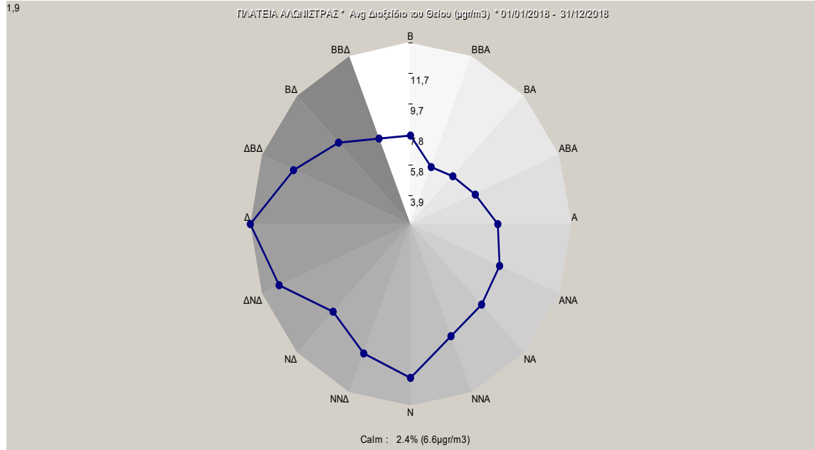
Σχήμα 3.3.: Μέσες τιμές διοξειδίου του θείου (σε \mu\text{g}/\text{m}^3 ) για κάθε διεύθυνση του ανέμου, για το έτος 2018.
