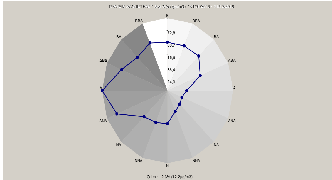
Σχήμα 3.4.: Μέσες τιμές όζοντος (σε \mu\text{g}/\text{m}^3 ) για κάθε διεύθυνση του ανέμου, για το έτος 2018.
