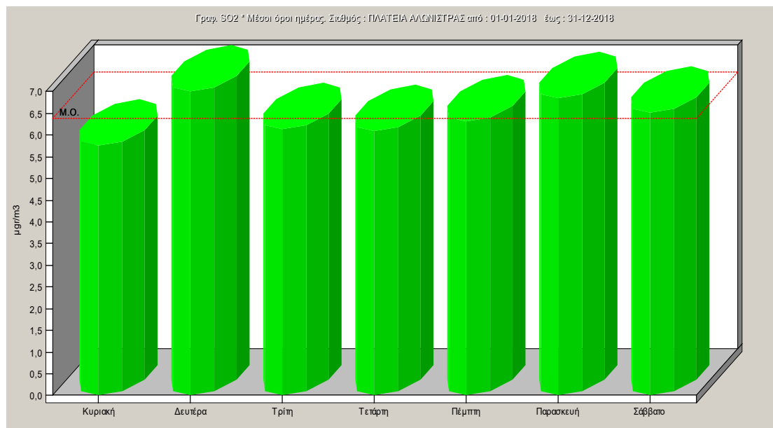
Σχήμα 2.11: Ημερήσια μεταβολή των συγκεντρώσεων διοξειδίου του θείου για το έτος 2018.
