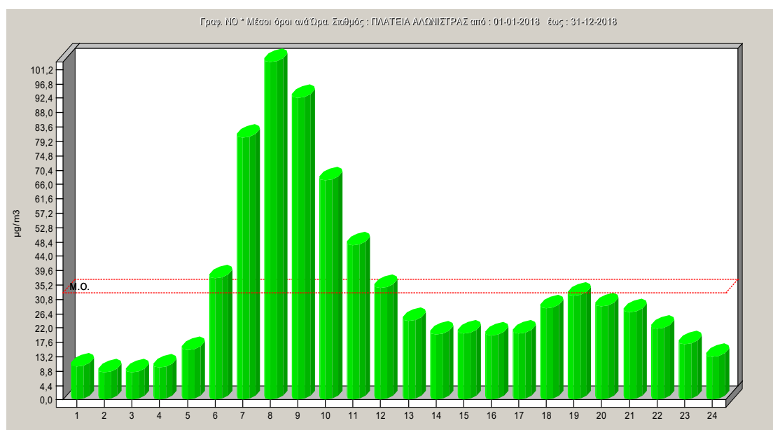
Σχήμα 2.17: Ωριαία μεταβολή μονοξειδίου του αζώτου για το έτος 2018
