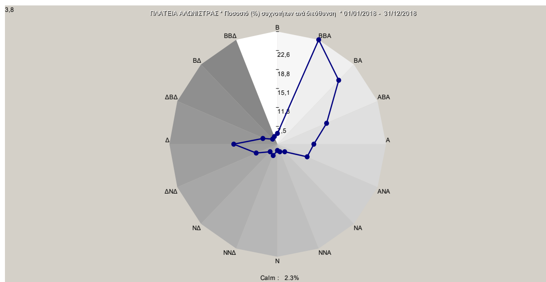
Σχήμα 3.1. Συχνότητες, επί τοις εκατό (%) των διευθύνσεων του ανέμου για το έτος 2018.
