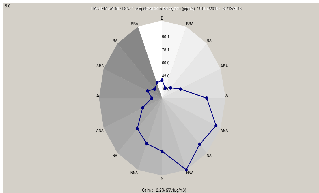
Σχήμα 3.5.: Μέσες τιμές μονοξειδίου του αζώτου, για κάθε διεύθυνση του ανέμου (σε \mu\text{g}/\text{m}^3 ), για το έτος 2018.
