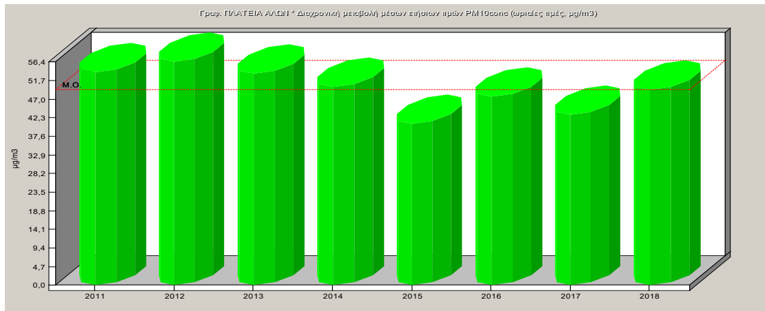
Σχήμα 2.5. Μέσες ετήσιες τιμές αιωρούμενων σωματιδίων 2011-2018.
