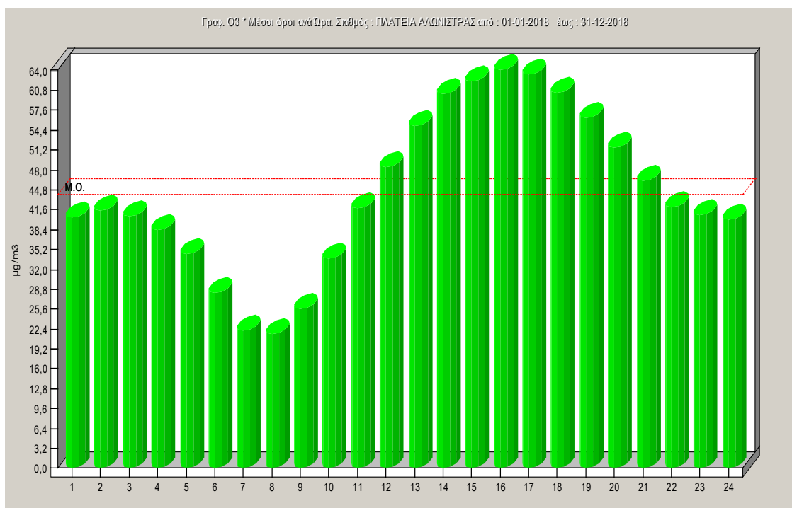
Σχήμα 2.19: Ωριαία μεταβολή όζοντος για το έτος 2018
