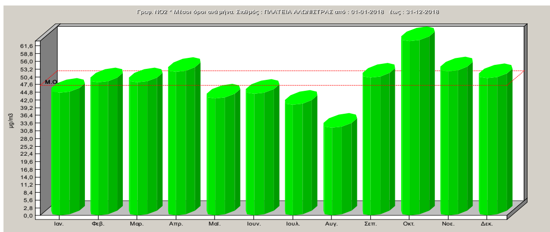
Σχήμα 2.8. Μέσες μηνιαίες τιμές διοξειδίου του αζώτου για το έτος 2018.
