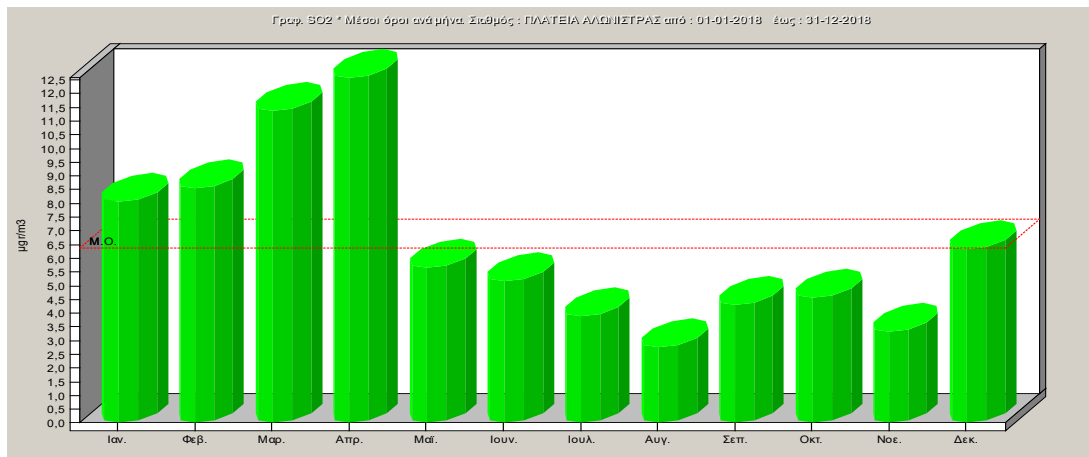
Σχήμα 2.6. Μέσες μηνιαίες τιμές διοξειδίου του θείου για το έτος 2018.
