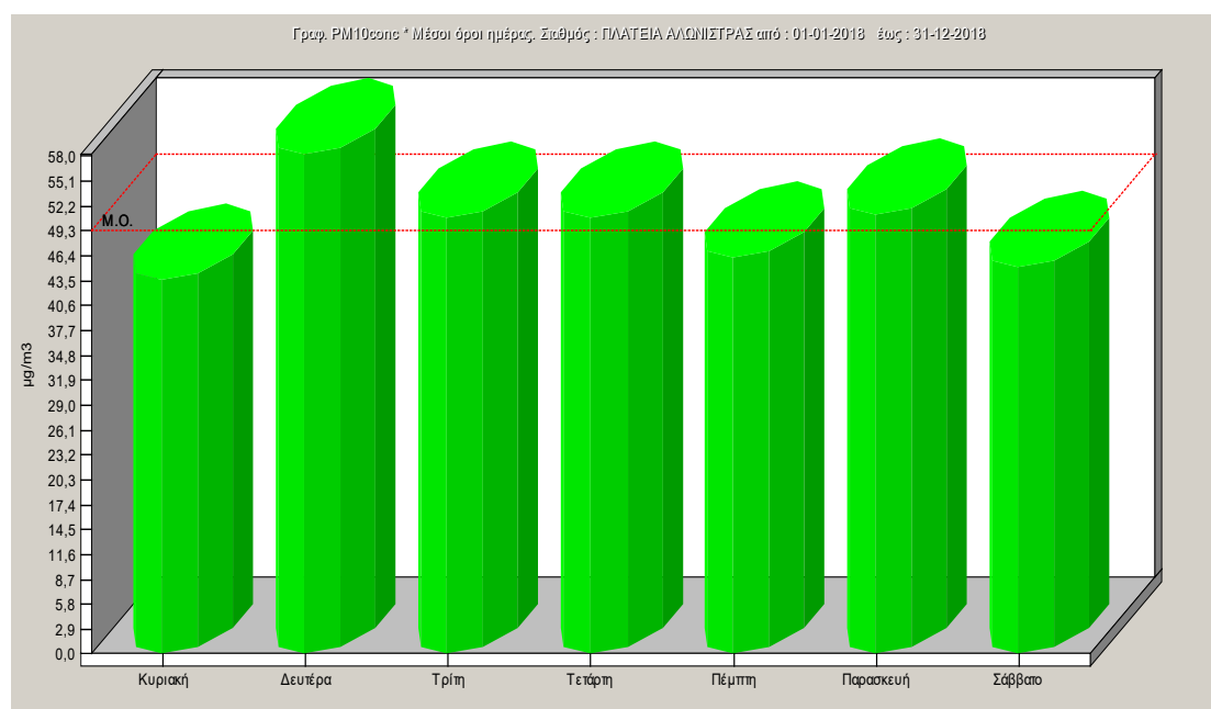
Σχήμα 2.15: Ημερήσια μεταβολή των συγκεντρώσεων αιωρούμενων σωματιδίων για το έτος 2018.
