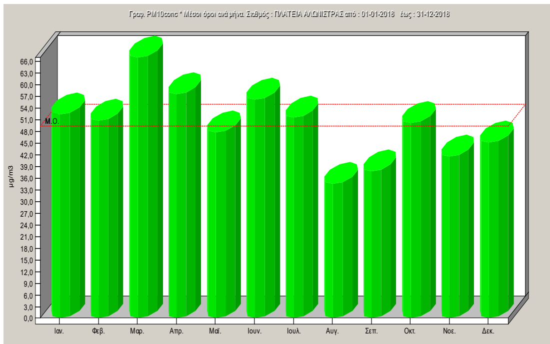
Σχήμα 2.10. Μέσες μηνιαίες τιμές αιωρούμενων σωματιδίων για το έτος 2018.
