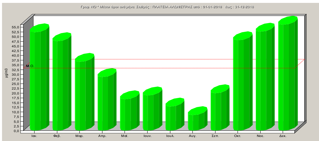
Σχήμα 2.7. Μέσες μηνιαίες τιμές μονοξειδίου του αζώτου για το έτος 2018.
