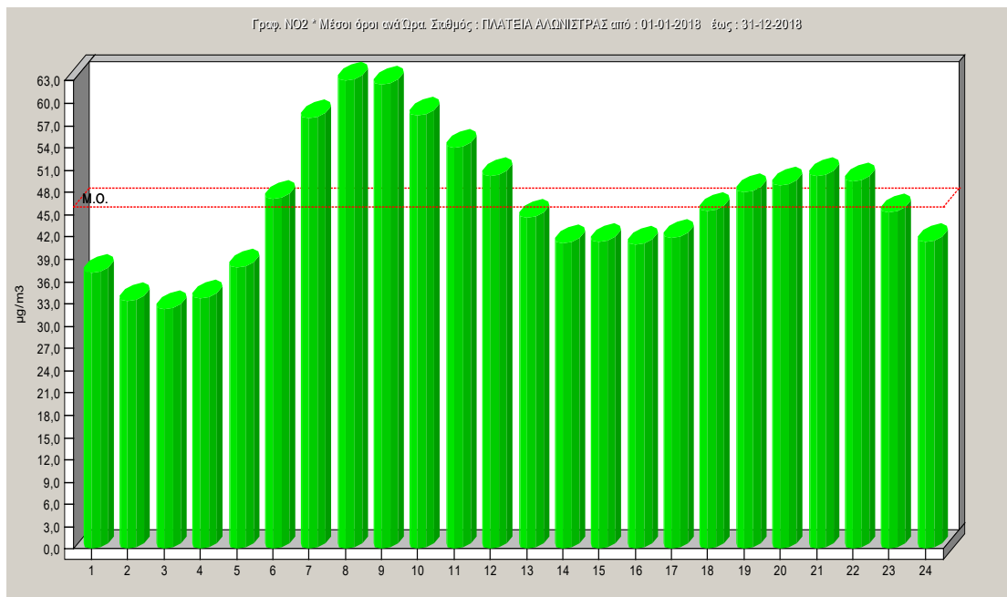
Σχήμα 2.18: Ωριαία μεταβολή διοξειδίου του αζώτου για το έτος 2018
