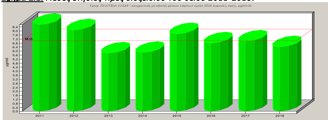
Σχήμα 2.1. Μέσες ετήσιες τιμές διοξειδίου του θείου 2011-2018.
