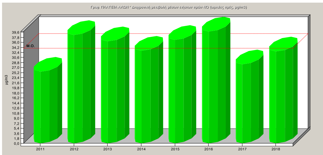
Σχήμα 2.2. Μέσες ετήσιες τιμές μονοξειδίου του αζώτου 2011-2018.
