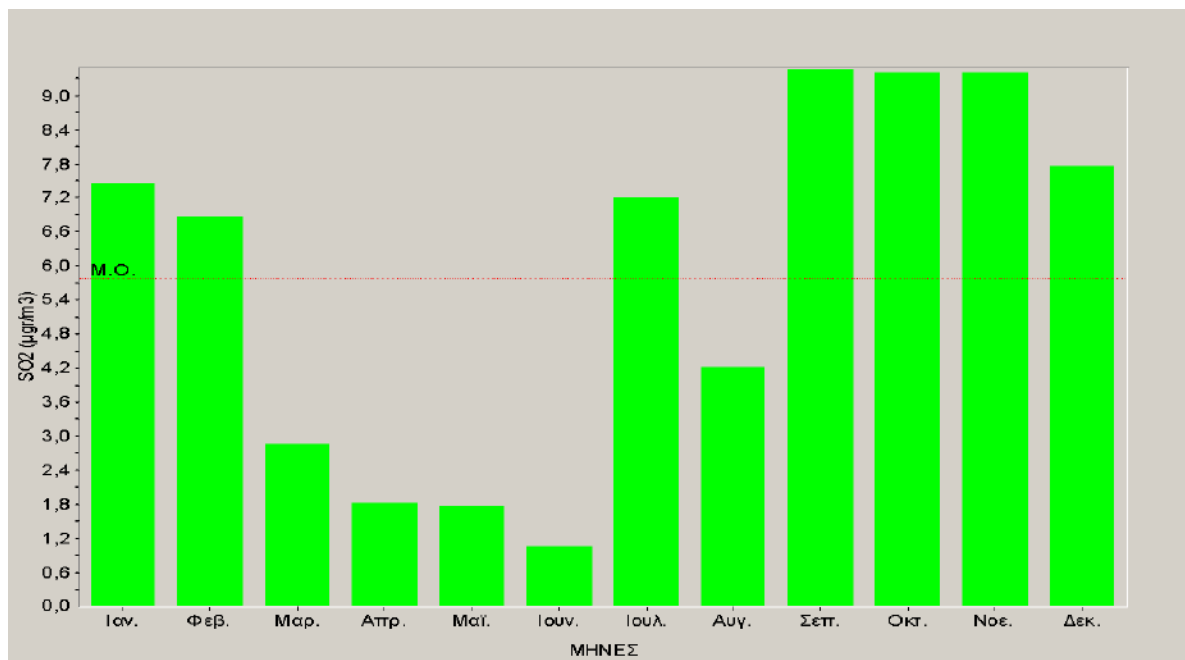
Σχήμα 2.1. Μέσες μηνιαίες τιμές διοξειδίου του θείου για το έτος 2013.
