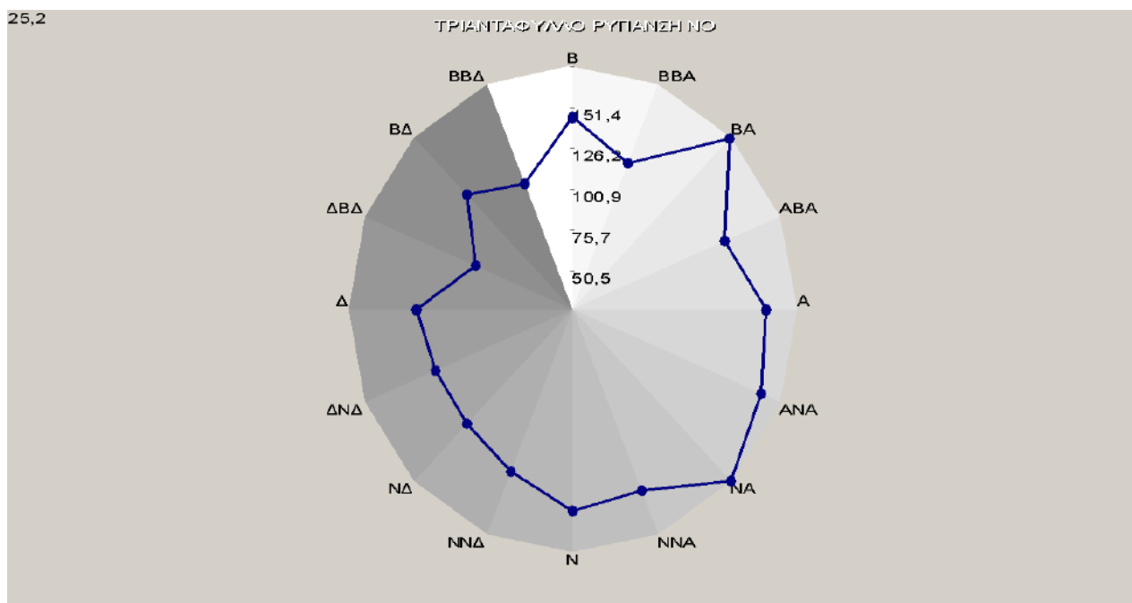
Σχήμα 3.5.: Μέσες τιμές μονοξειδίου του αζώτου, για κάθε διεύθυνση του ανέμου (σε \mu\text{g}/\text{m}^3 ), για το έτος 2013.
