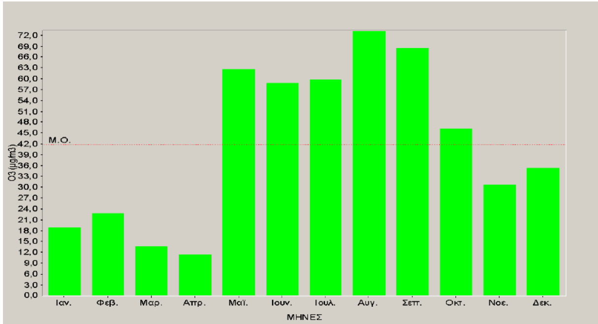
Σχήμα 2.2. Μέσες μηνιαίες τιμές όζοντος για το έτος 2013.
