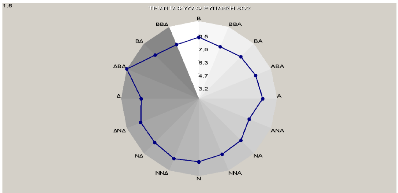
Σχήμα 3.3.: Μέσες τιμές διοξειδίου του θείου (σε \mu\text{g}/\text{m}^3 ) για κάθε διεύθυνση του ανέμου, για το έτος 2013.
