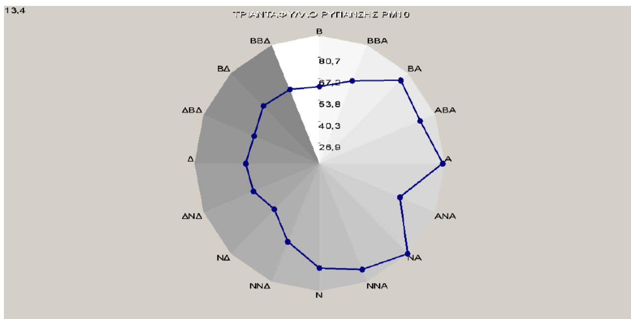
Σχήμα 3.7.: Μέσες τιμές Αιωρούμενων Σωματιδίων (σε \mu\text{g}/\text{m}^3 ), για κάθε διεύθυνση του ανέμου, για το έτος 2013.
