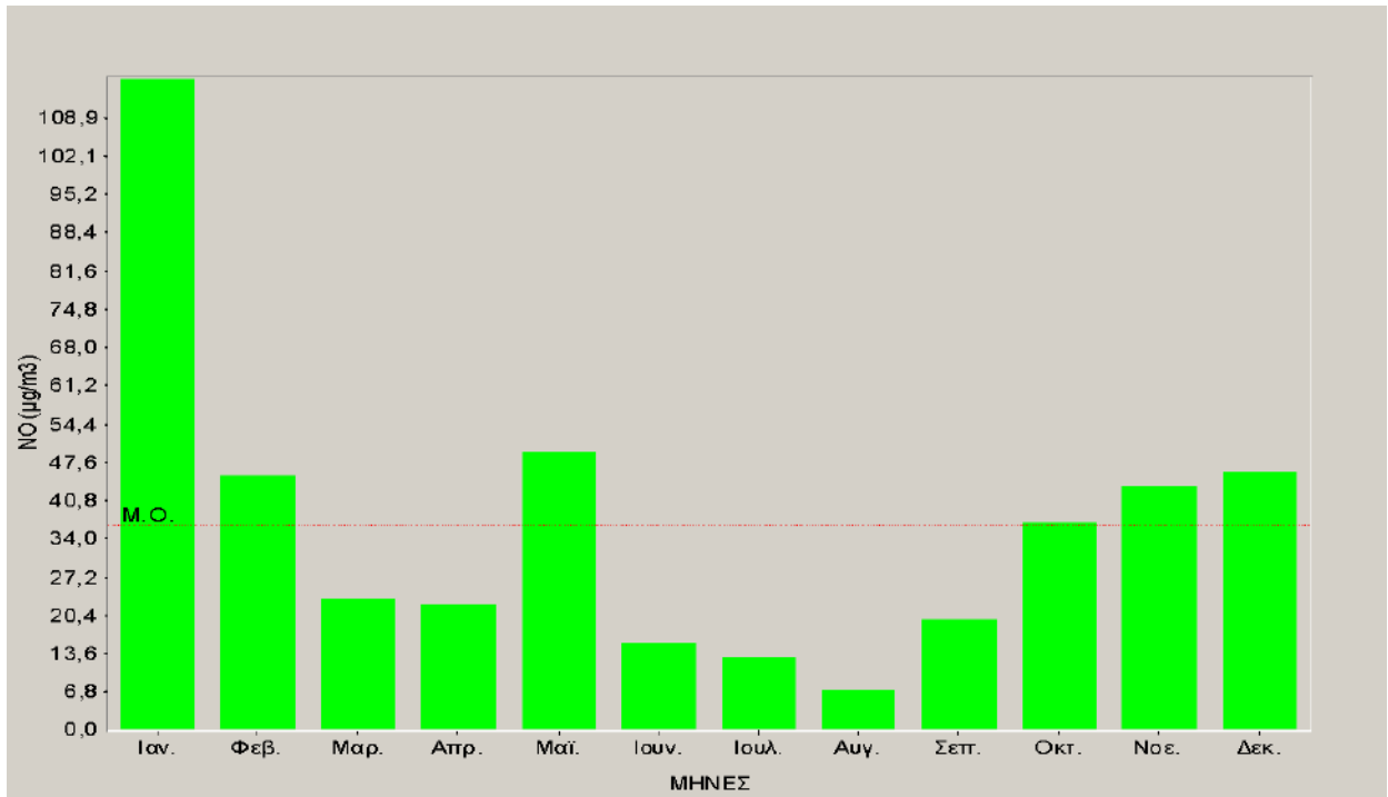
Σχήμα 2.3. Μέσες μηνιαίες τιμές μονοξειδίου του αζώτου για το έτος 2013.
