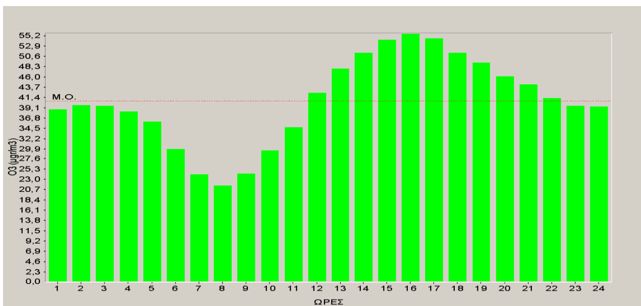
Σχήμα 2.12: Ωριαία μεταβολή όζοντος για το έτος 2013
