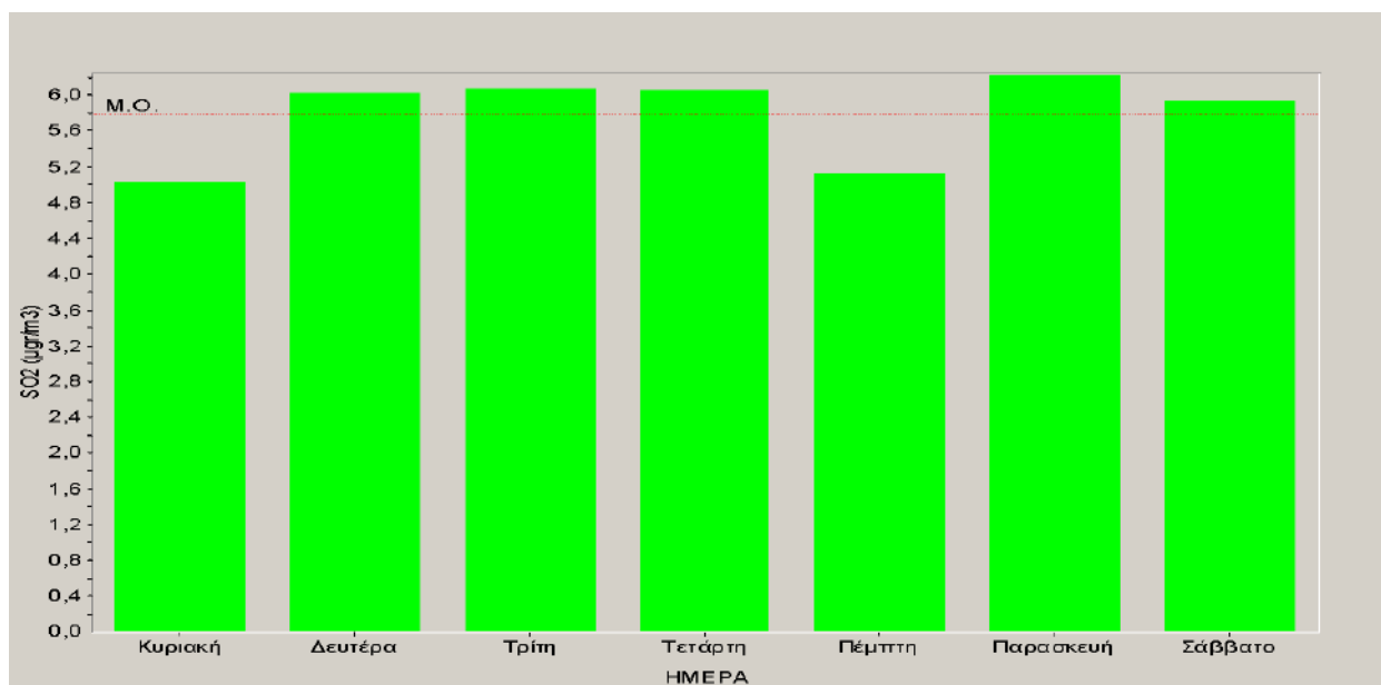
Σχήμα 2.6: Ημερήσια μεταβολή των συγκεντρώσεων διοξειδίου του θείου για το έτος 2013.
