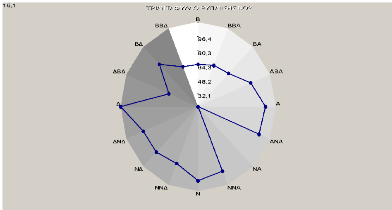
Σχήμα 3.6.: Μέσες τιμές διοξειδίου του αζώτου (σε \mu\text{g}/\text{m}^3 ), για κάθε διεύθυνση του ανέμου, για το έτος 2013.
