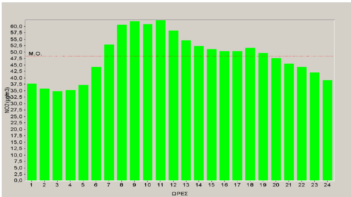
Σχήμα 2.14: Ωριαία μεταβολή διοξειδίου του αζώτου για το έτος 2013
