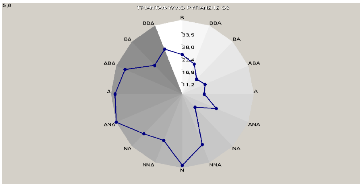
Σχήμα 3.4.: Μέσες τιμές όζοντος (σε \mu\text{g}/\text{m}^3 ) για κάθε διεύθυνση του ανέμου, για το έτος 2013.
