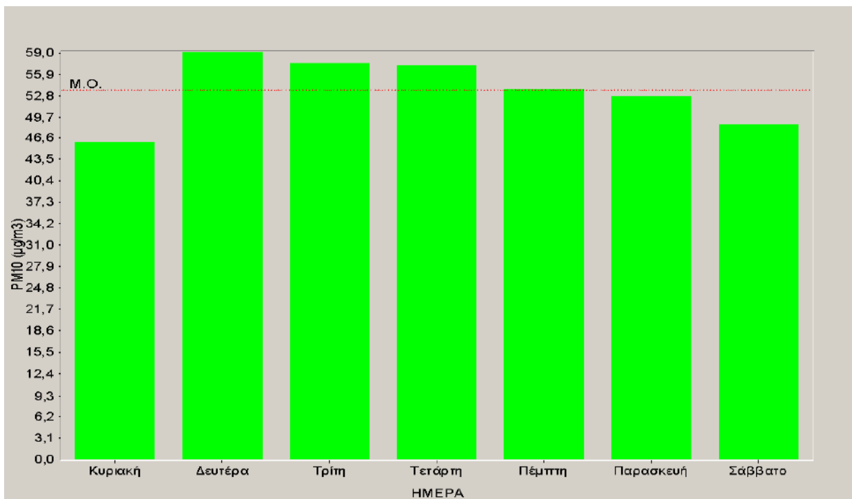
Σχήμα 2.10: Ημερήσια μεταβολή των συγκεντρώσεων αιωρούμενων σωματιδίων για το έτος 2013.
