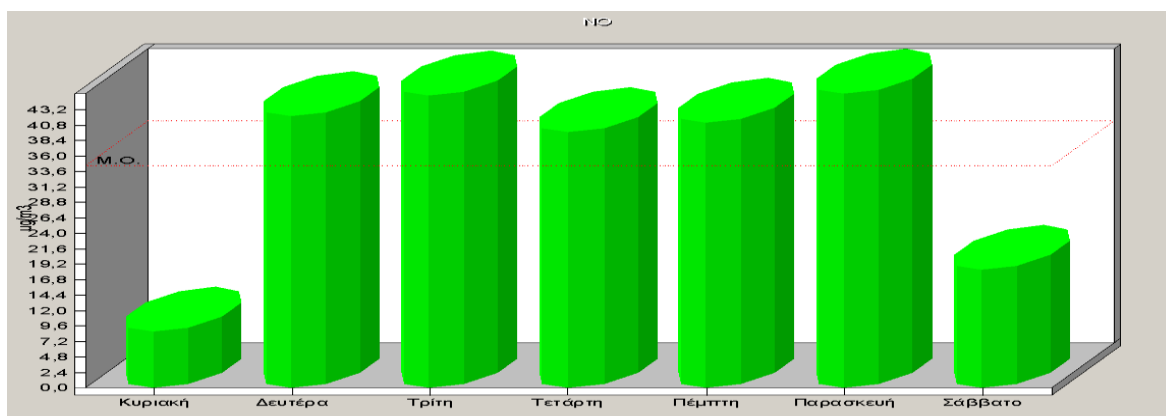
Σχήμα 2.14: Ημερήσια μεταβολή των συγκεντρώσεων μονοξειδίου του αζώτου για το έτος 2024.
