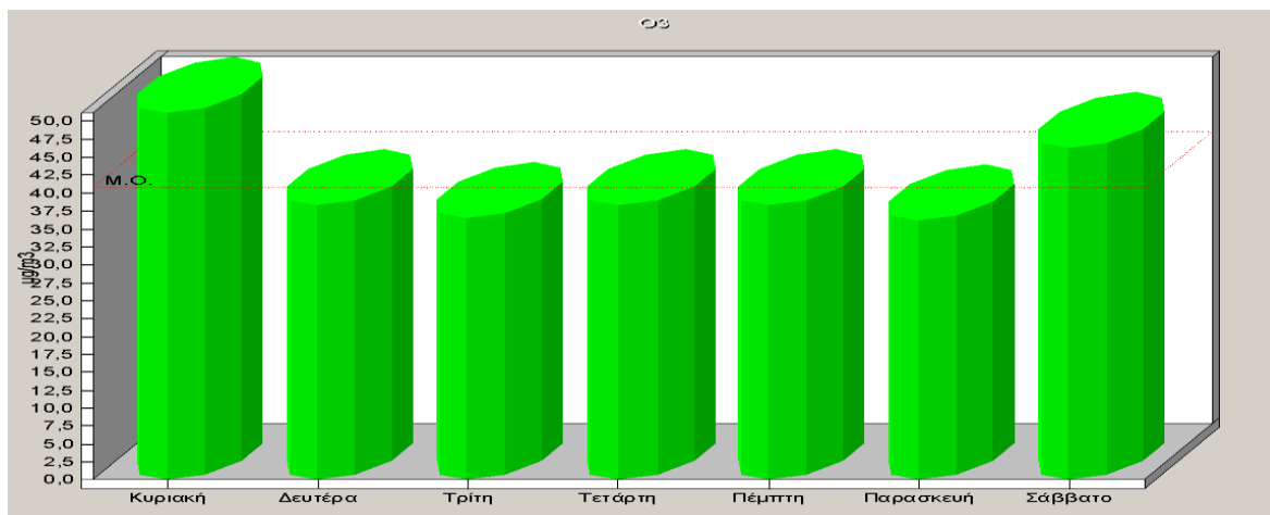
Σχήμα 2.16: Ημερήσια μεταβολή των συγκεντρώσεων όζοντος για το έτος 2024.
