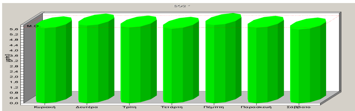
Σχήμα 2.13: Ημερήσια μεταβολή των συγκεντρώσεων διοξειδίου του θείου για το έτος 2024.
