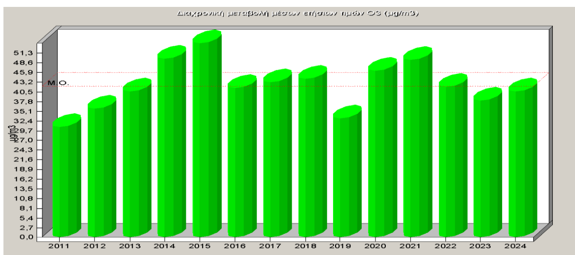
Σχήμα 2.4. Μέσες ετήσιες τιμές όζοντος 2011-2024.
