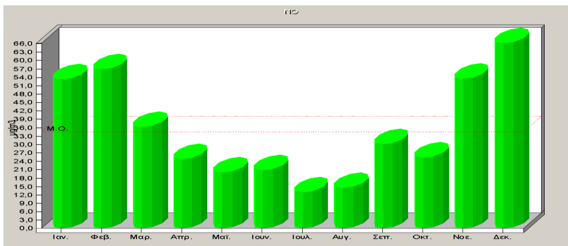
Σχήμα 2.8. Μέσες μηνιαίες τιμές μονοξειδίου του αζώτου για το έτος 2024.
