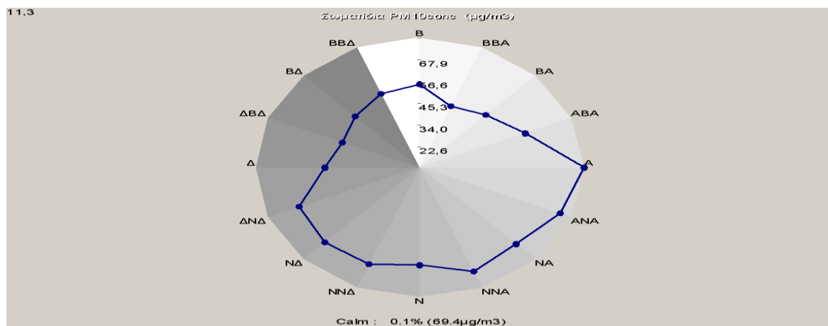
Σχήμα 3.7.: Μέσες τιμές Αιωρουμένων Σωματιδίων (PM10) (σε \mu\text{g}/\text{m}^3 ), για κάθε διεύθυνση του ανέμου, για το έτος 2024.
