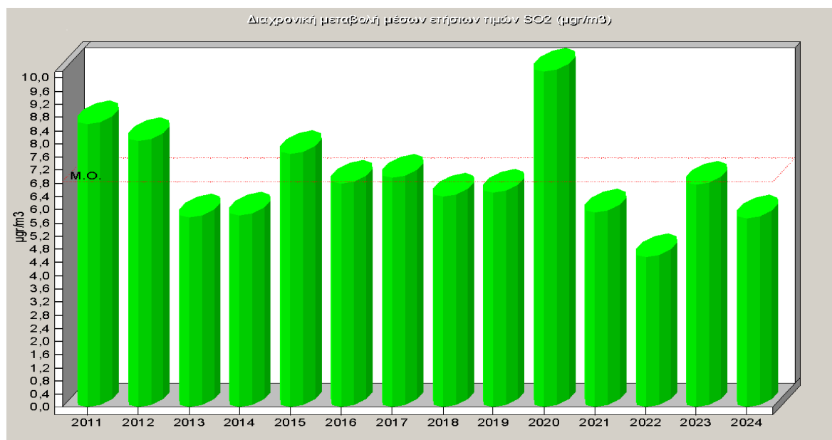
Σχήμα 2.1. Μέσες ετήσιες τιμές διοξειδίου του θείου 2011-2024.
