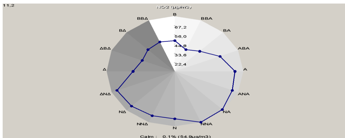
Σχήμα 3.6.: Μέσες τιμές διοξειδίου του αζώτου (σε \mu\text{g}/\text{m}^3 ), για κάθε διεύθυνση του ανέμου, για το έτος 2024.
