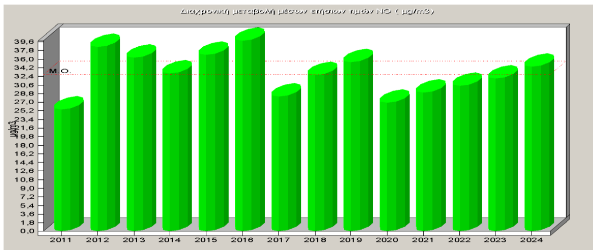
Σχήμα 2.2. Μέσες ετήσιες τιμές μονοξειδίου του αζώτου 2011-2024.
