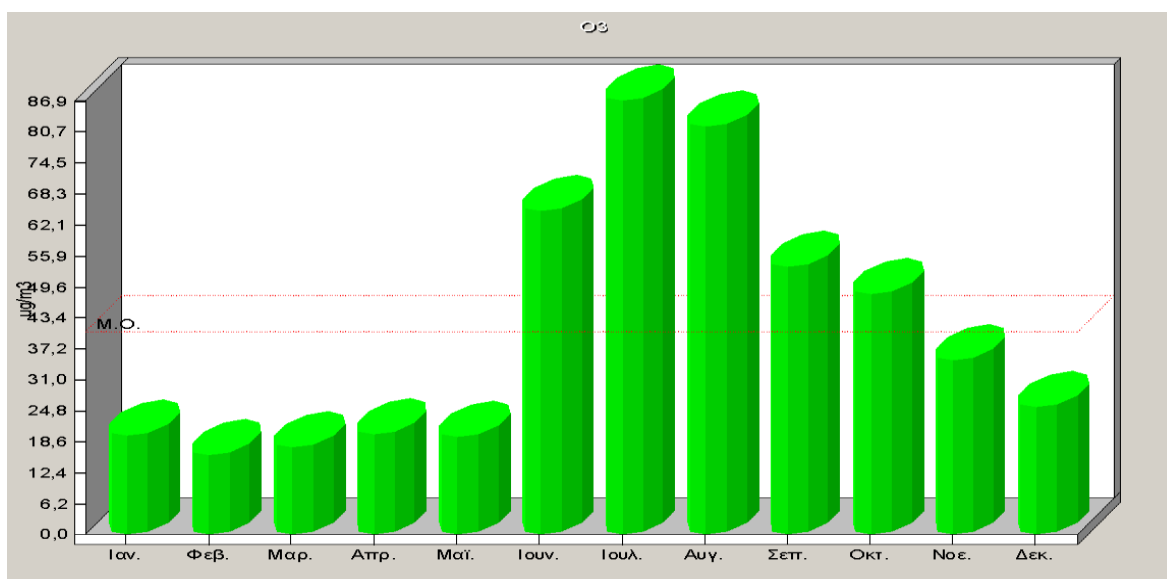
Σχήμα 2.10. Μέσες μηνιαίες τιμές όζοντος για το έτος 2024.
