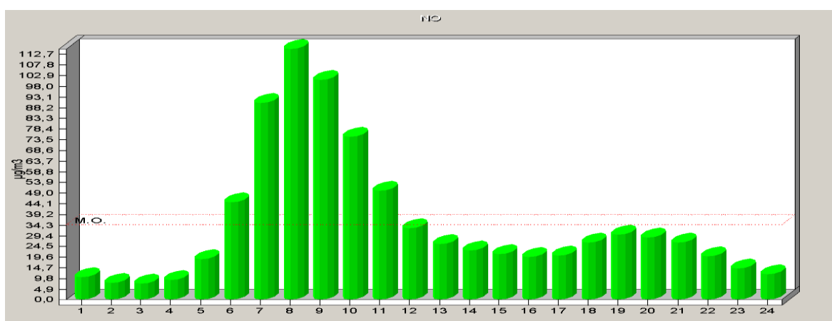
Σχήμα 2.20: Ωριαία μεταβολή μονοξειδίου του αζώτου για το έτος 2024.
