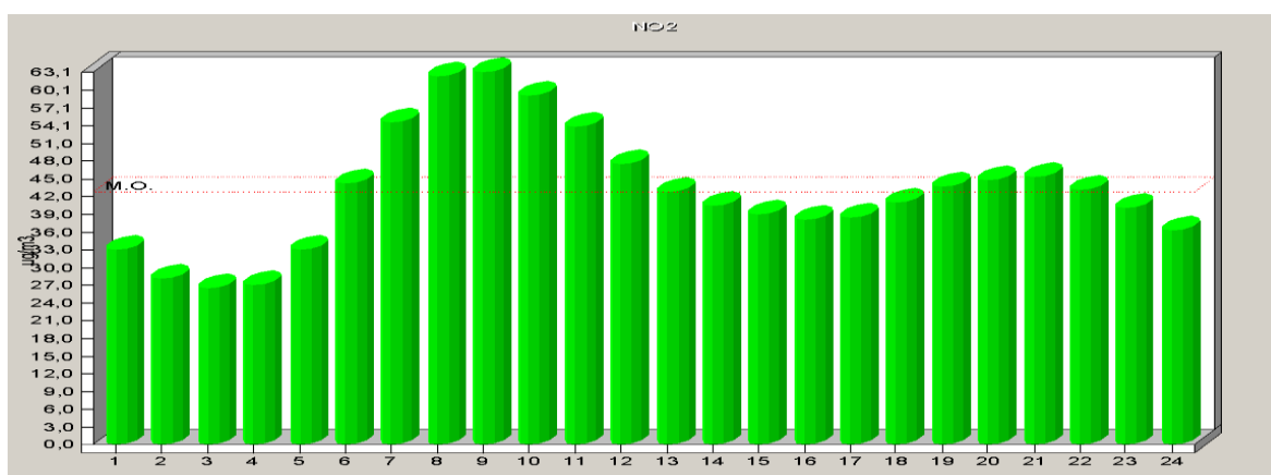
Σχήμα 2.21: Ωριαία μεταβολή διοξειδίου του αζώτου για το έτος 2024.
