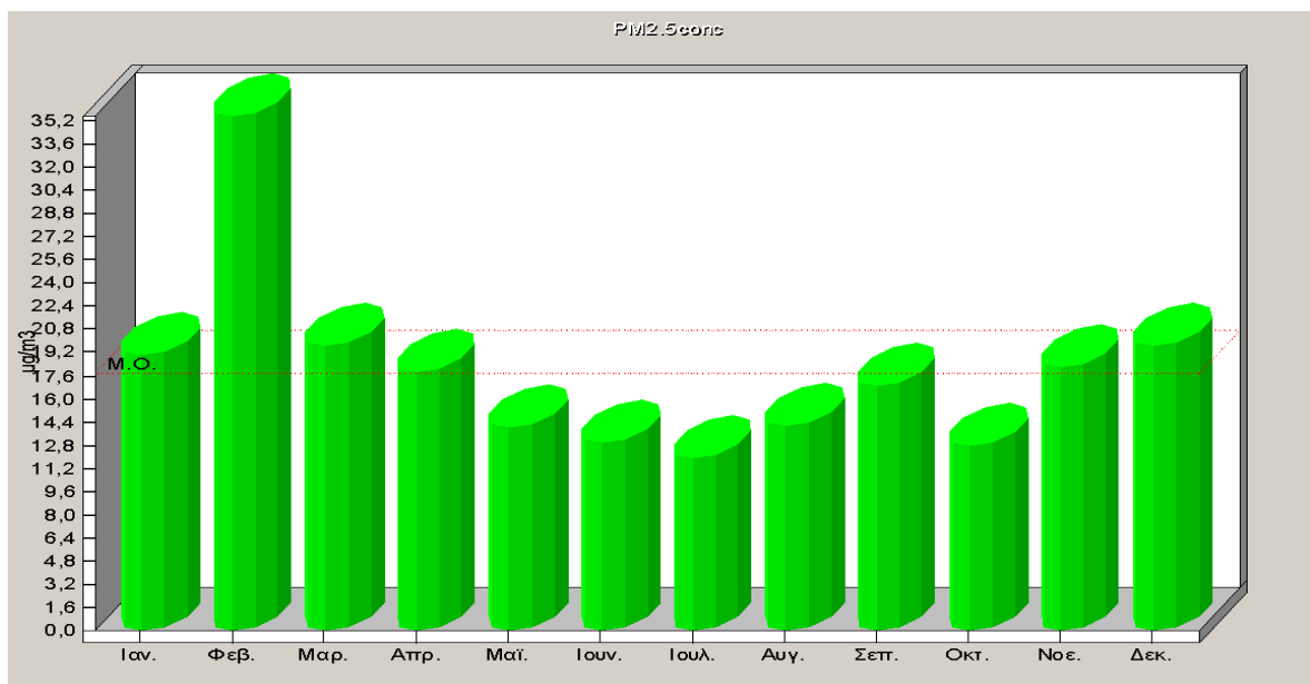
Σχήμα 2.12. Μέσες μηνιαίες τιμές αιωρούμενων σωματιδίων (PM2.5) για το έτος 2024.
