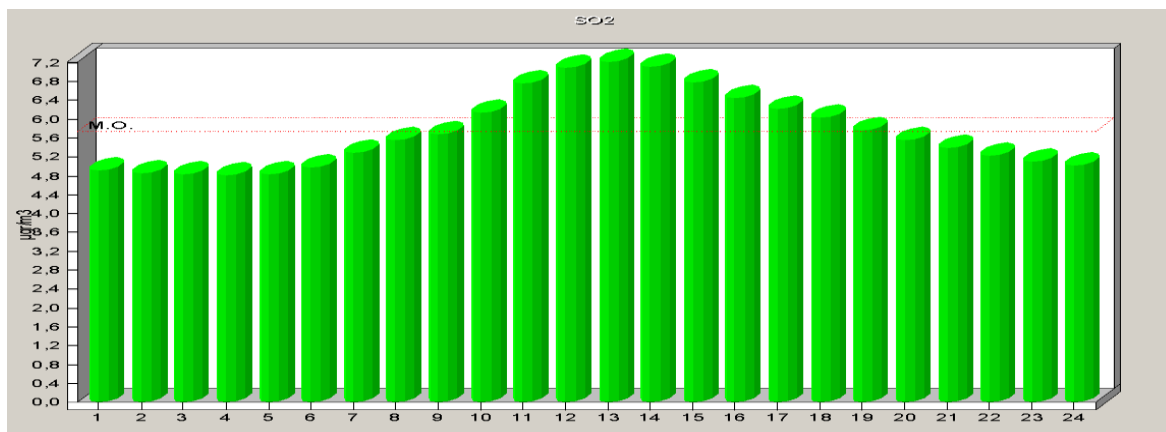
Σχήμα 2.19: Ωριαία μεταβολή διοξειδίου του θείου για το έτος 2024.
