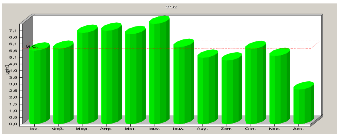
Σχήμα 2.7. Μέσες μηνιαίες τιμές διοξειδίου του θείου για το έτος 2024.
