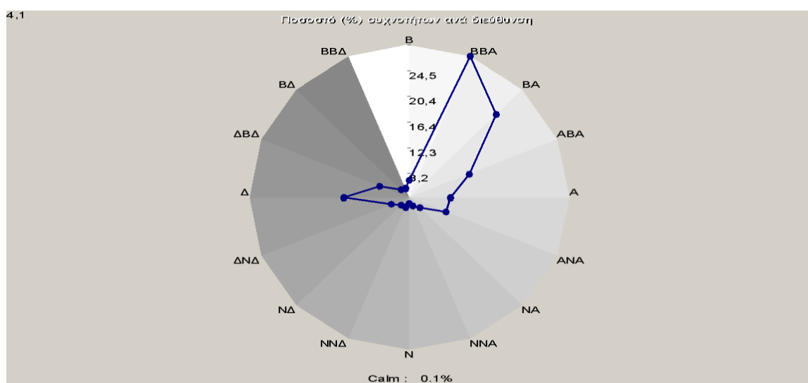
Σχήμα 3.1. Συχνότητες, επί τοις εκατό (%) των διευθύνσεων του ανέμου για το έτος 2024.
