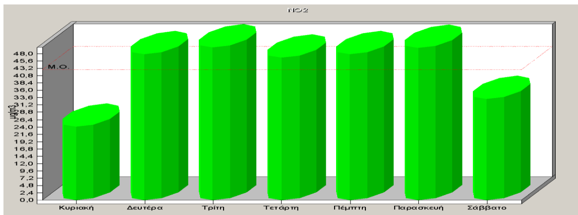
Σχήμα 2.15: Ημερήσια μεταβολή των συγκεντρώσεων διοξειδίου του αζώτου για το έτος 2024.
