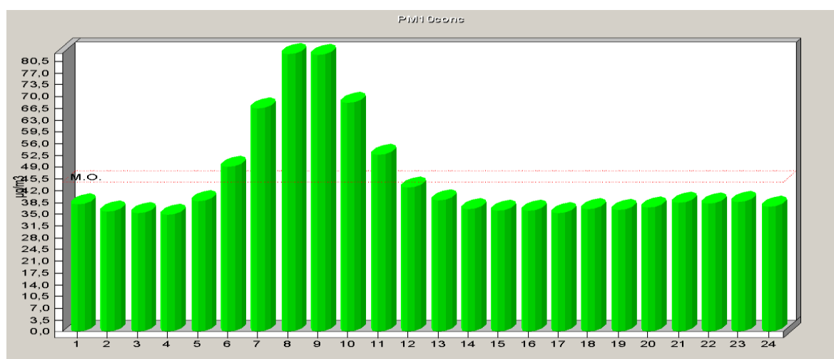
Σχήμα 2.23: Ωριαία μεταβολή αιωρούμενων σωματιδίων (PM10) για το έτος 2024.
