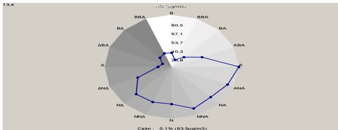
Σχήμα 3.5.: Μέσες τιμές μονοξειδίου του αζώτου, για κάθε διεύθυνση του ανέμου (σε \mu\text{g}/\text{m}^3 ), για το έτος 2024.
