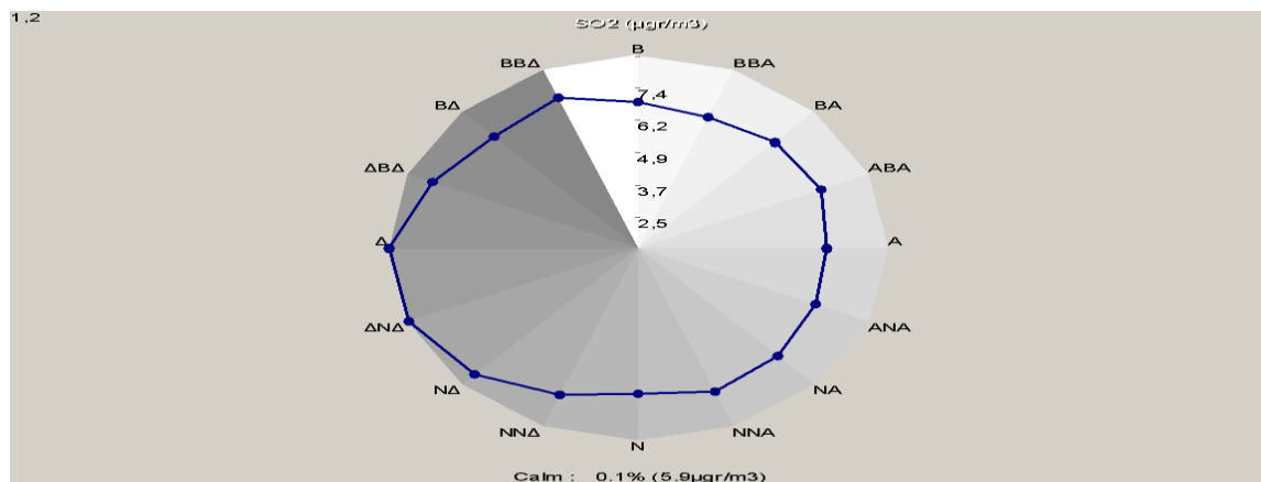
Σχήμα 3.3.: Μέσες τιμές διοξειδίου του θείου (σε \mu\text{g}/\text{m}^3 ), για κάθε διεύθυνση του ανέμου, για το έτος 2024.
