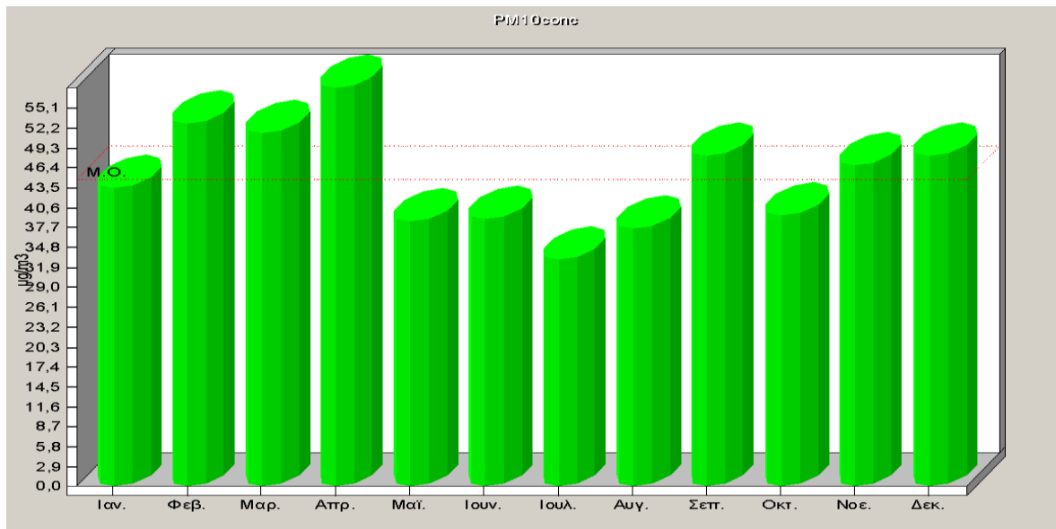
Σχήμα 2.11. Μέσες μηνιαίες τιμές αιωρούμενων σωματιδίων (PM10) για το έτος 2024.
