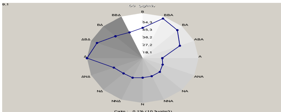
Σχήμα 3.4.: Μέσες τιμές όζοντος (σε \mu\text{g}/\text{m}^3 ), για κάθε διεύθυνση του ανέμου, για το έτος 2024.
