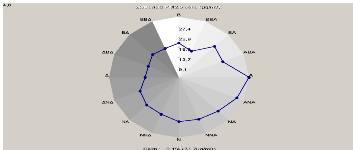
Σχήμα 3.8.: Μέσες τιμές Αιωρουμένων Σωματιδίων (PM2.5) (σε \mu\text{g}/\text{m}^3 ), για κάθε διεύθυνση του ανέμου, για το έτος 2024.
