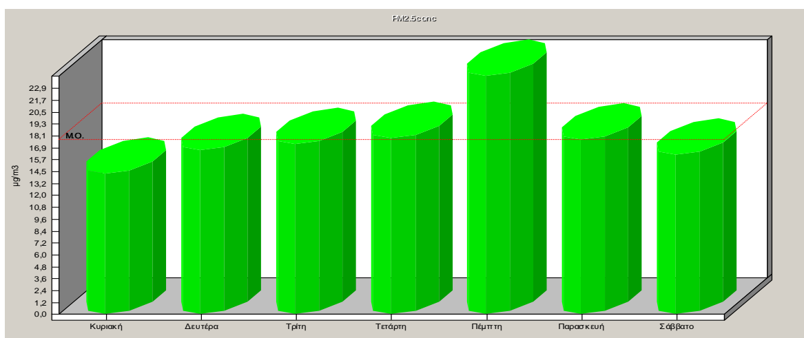
Σχήμα 2.18: Ημερήσια μεταβολή των συγκεντρώσεων αιωρούμενων σωματιδίων (PM2.5) για το έτος 2024.
