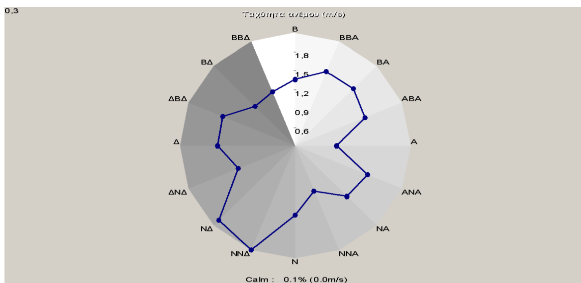
Σχήμα 3.2 Μέση ταχύτητα ανά διεύθυνση ανέμου, για το έτος 2024.
