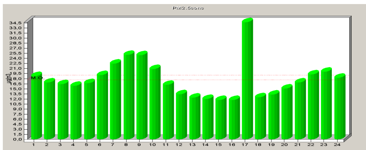
Σχήμα 2.24: Ωριαία μεταβολή αιωρούμενων σωματιδίων (PM2.5) για το έτος 2024.
