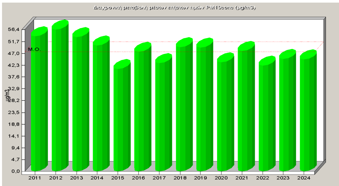
Σχήμα 2.5. Μέσες ετήσιες τιμές αιωρούμενων σωματιδίων (PM10) 2011-2024.
