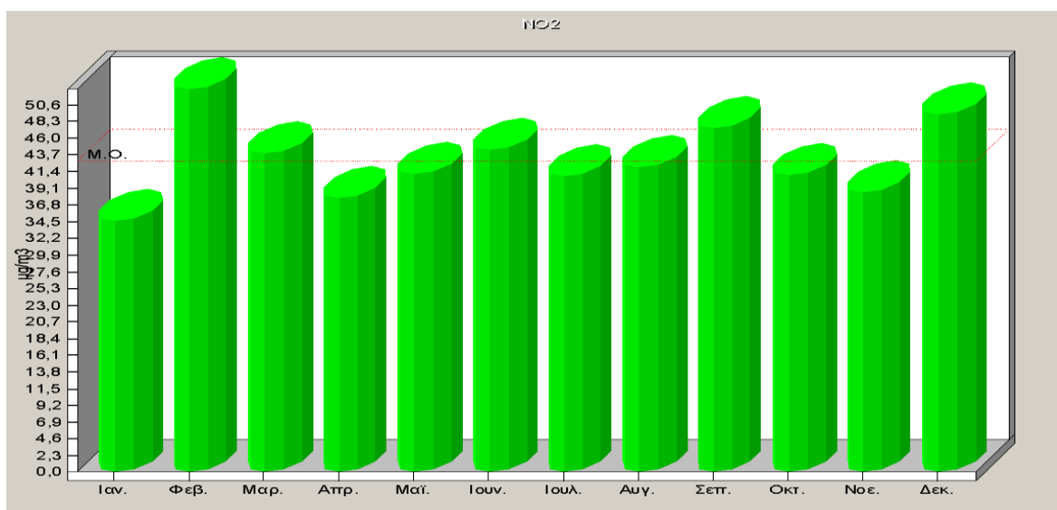
Σχήμα 2.9. Μέσες μηνιαίες τιμές διοξειδίου του αζώτου για το έτος 2024.
