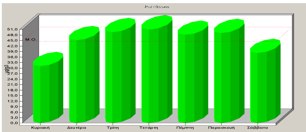
Σχήμα 2.17: Ημερήσια μεταβολή των συγκεντρώσεων αιωρούμενων σωματιδίων (PM10) για το έτος 2024.
