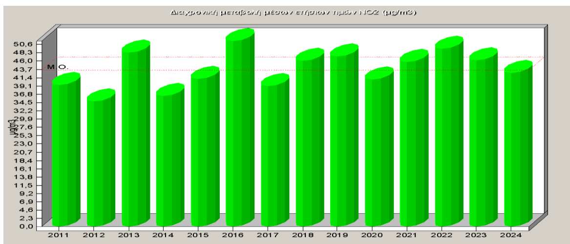
Σχήμα 2.3. Μέσες ετήσιες τιμές διοξειδίου του αζώτου 2011-2024.
