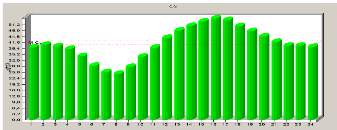
Σχήμα 2.22: Ωριαία μεταβολή όζοντος για το έτος 2024.
